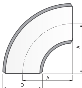
90° LONG RADIUS ELBOW
