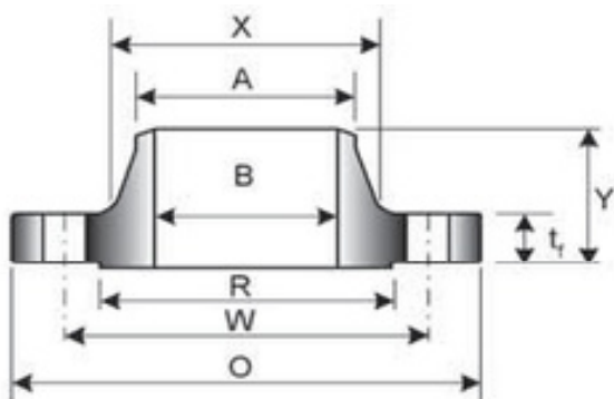
Vorschweißflansch / Welding Neck Flange
