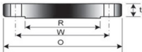
Blindflansch / Blind Flange
