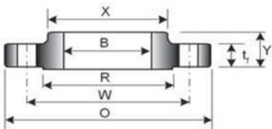
Überschiebschweißflansch / Slip-On Flange
