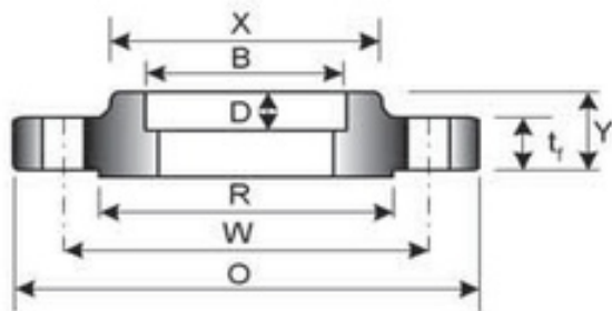
Einsteckschweißflansch / Socket Welding Flange
