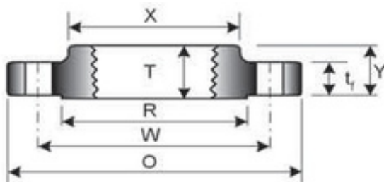
Gewindeflansch / Threaded Flange
